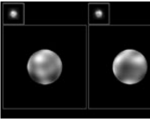
صور لسطح بلوتو من تلسكوب هبل مقارنة بالصور الملتقطة من المراصد الأرضية (في الأعلى)
